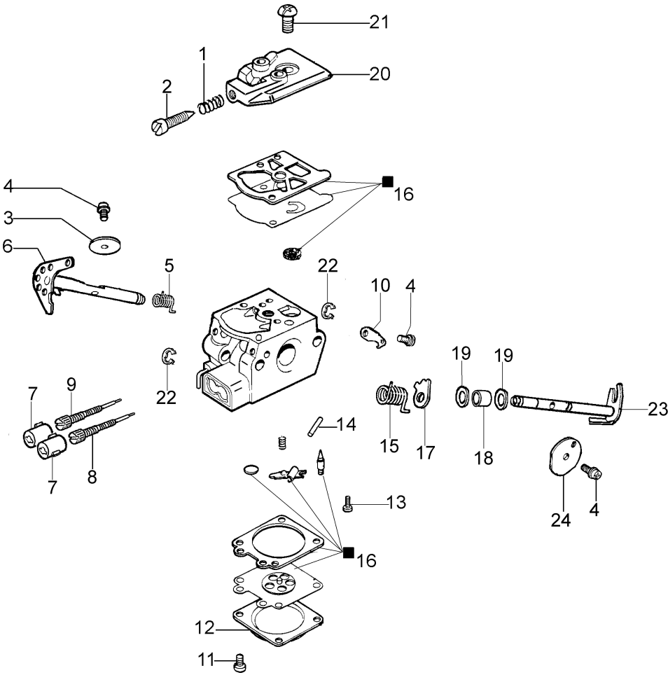
16 ■ KIT RIPARAZIONE REPAIR KIT
